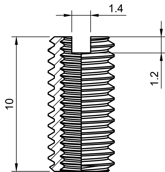
A-A
