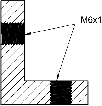
A-A
